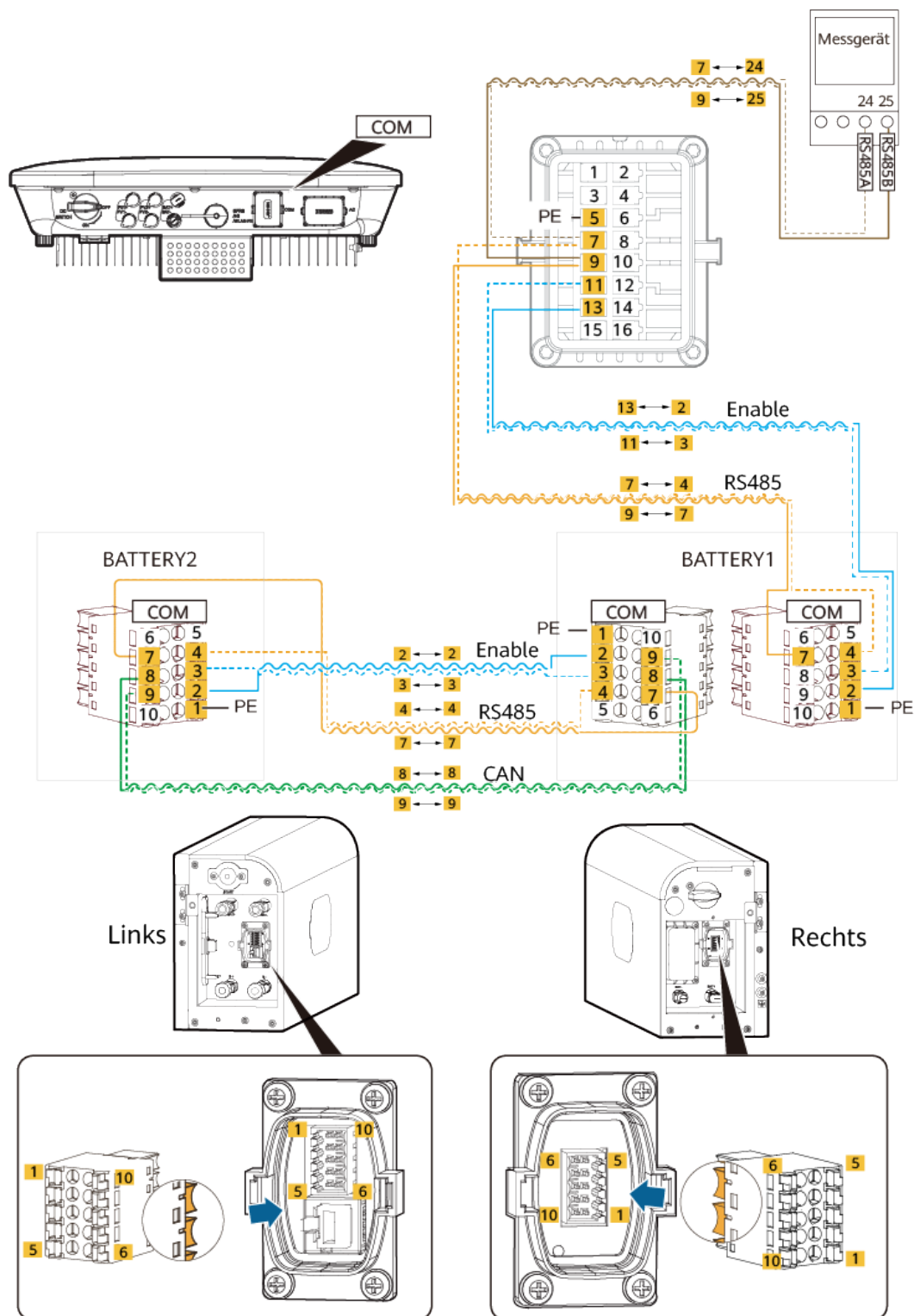
Abbildung 6-7 SUN2000-(3KTL-12KTL)-M1
