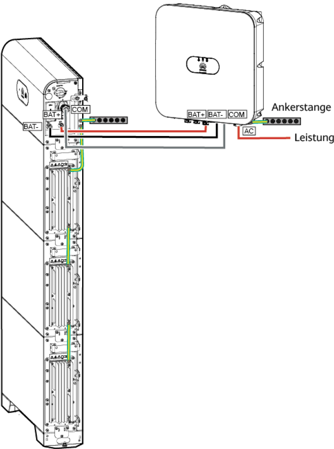
Abbildung 8-3 Kabelverbindungsplan
