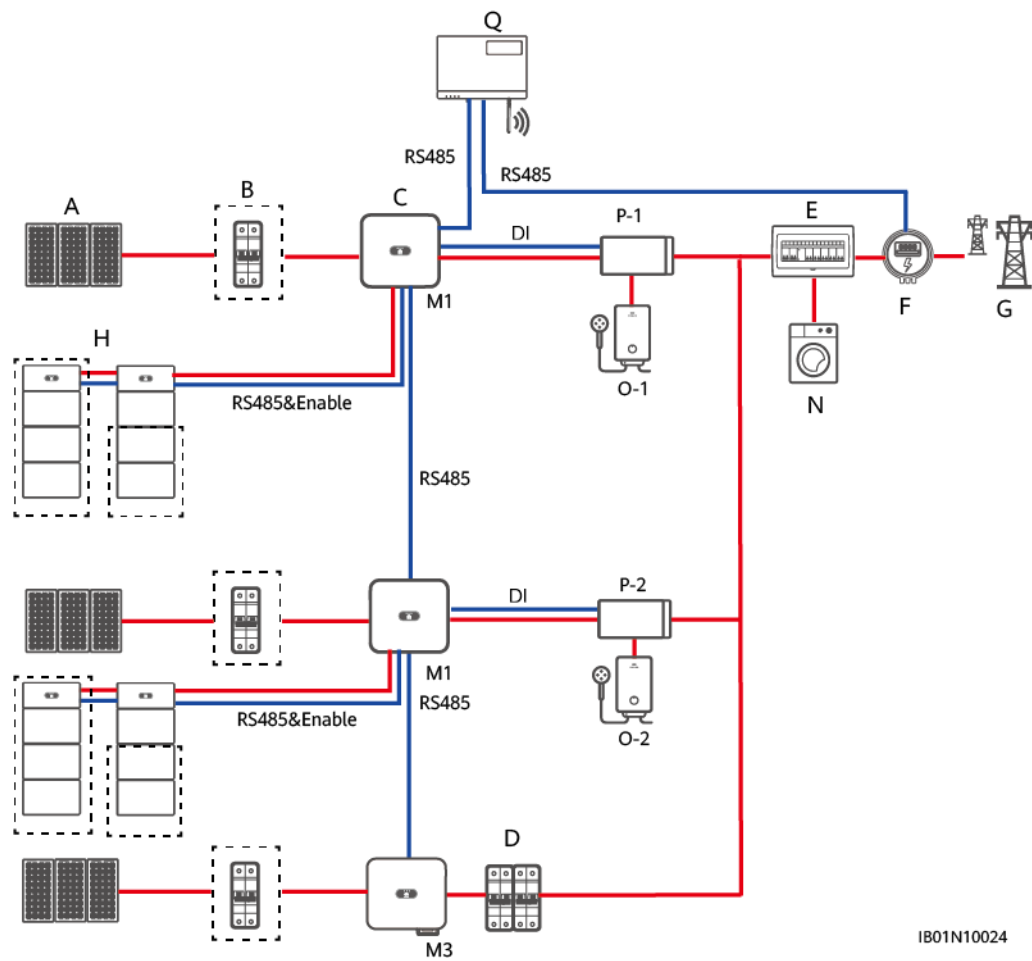
Abbildung 4-12 Vernetzung von zwei Wechselrichtern SUN2000-(3KTL-10KTL)-M1 mit einem Wechselrichter SUN2000-(20KTL, 29.9KTL, 30KTL, 36KTL, 40KTL)-M3 (gestrichelte Kästchen stehen für optionale Komponenten)
