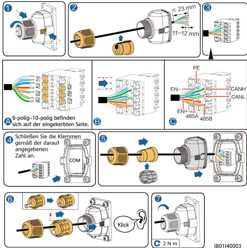
Abbildung 6-18 Kaskadierende Kommunikationsklemme
