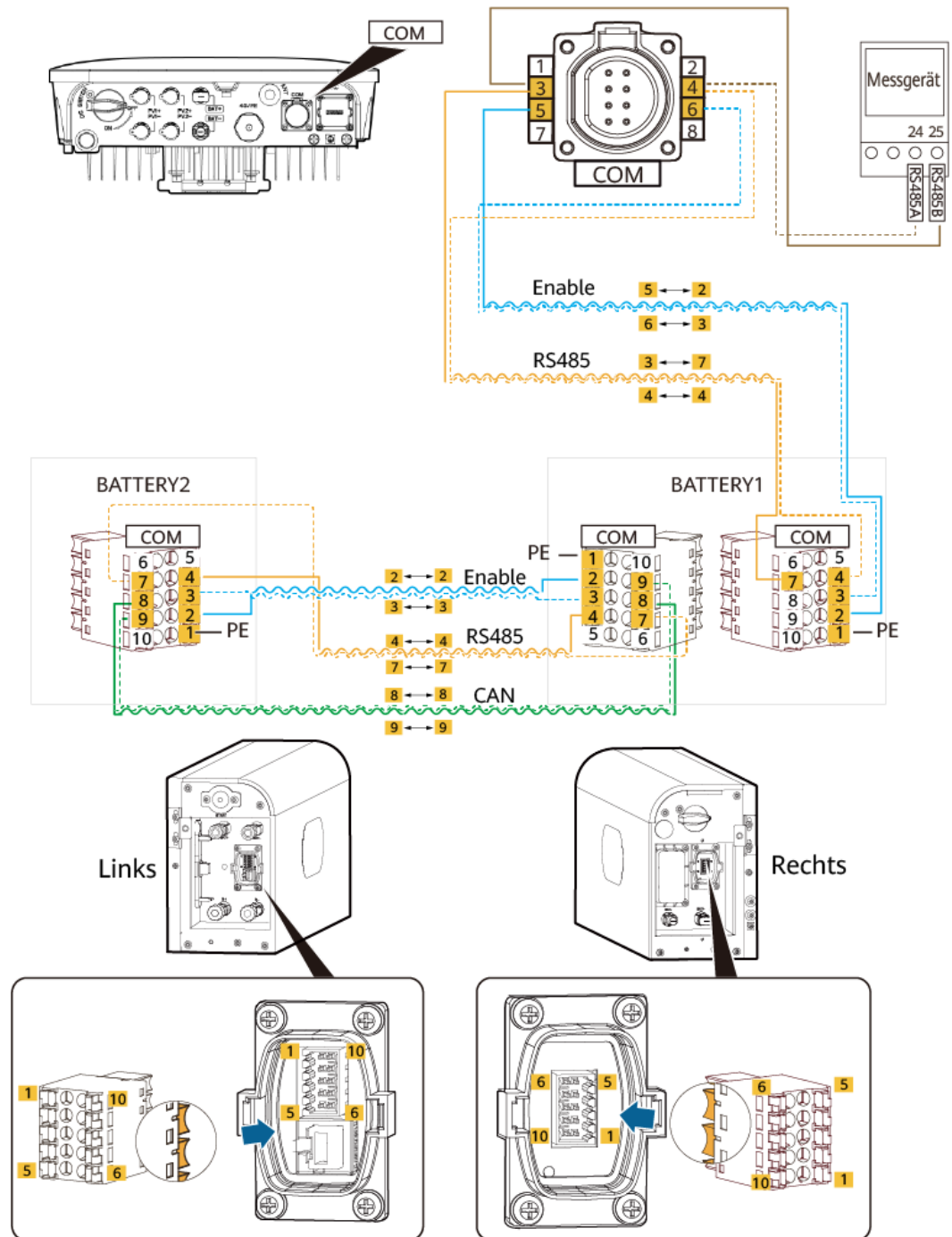
Abbildung 6-6 SUN2000-(2KTL-6KTL)-L1
