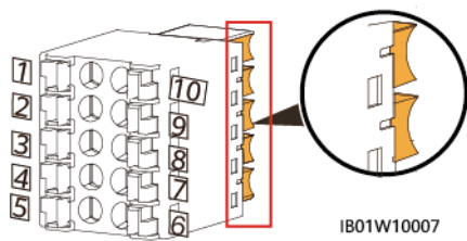
Abbildung 6-13 Signalkabelanschlüsse
