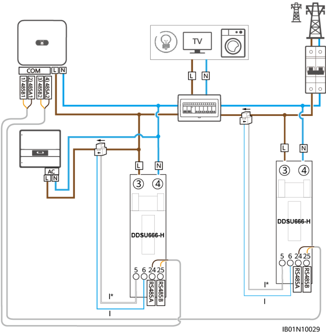
Abbildung 4-18 Kabelanschlüsse für Leistungsmesser an SUN2000-(2KTL-6KTL)-L1
