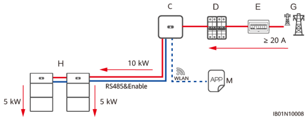
Abbildung 8-1 Netzwerkdiagramm für Szenario mit dreiphasiger Stromversorgung
